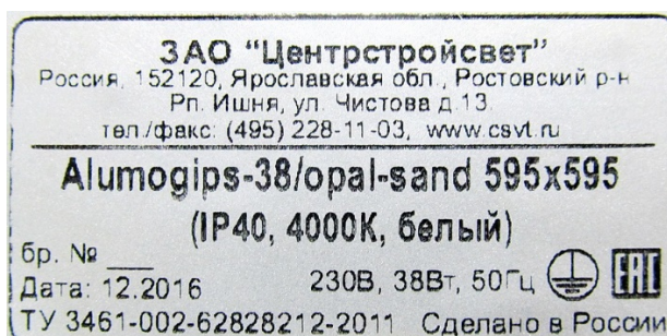
Светодиодный светильник ALIMOGIPS -38/opal sand 595x595 (IP40, 4000 К, белый) (Маркировка)
