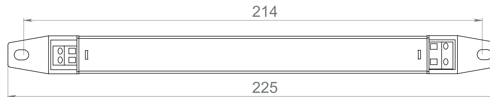
CSVT 54W-500mA-E-08
