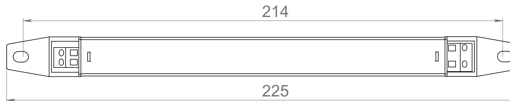
CSVT 54W-500mA-E-08
